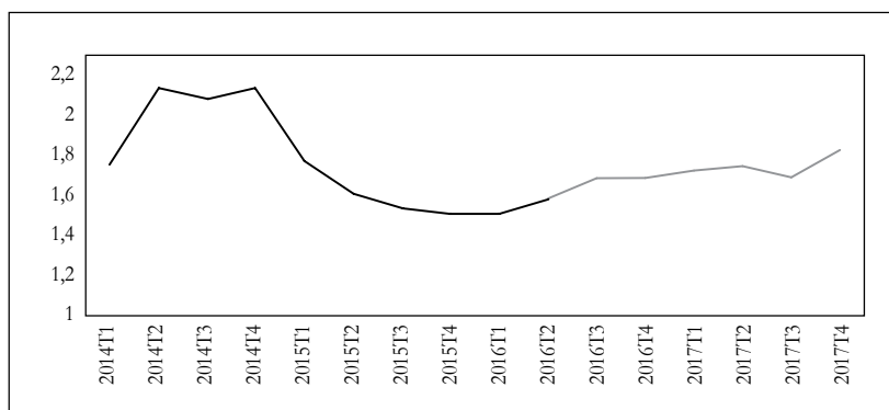
GRÁFICO 4.7 Los precios proyectados del café (USD por libra) 1/
